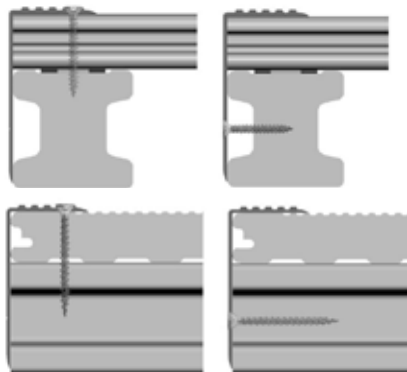
Avvitatura dall'alto
